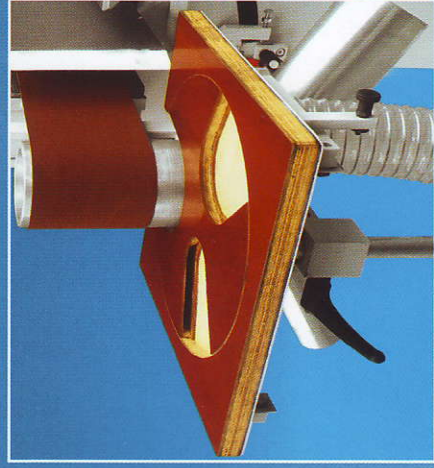
Въртяща се звезда с 2 контактни ролки (KSM 3000) Drehstern mit 2 zusätzlichen Kontaktwalzen (KSM 3000) Device STAR with 2 contact rollers
